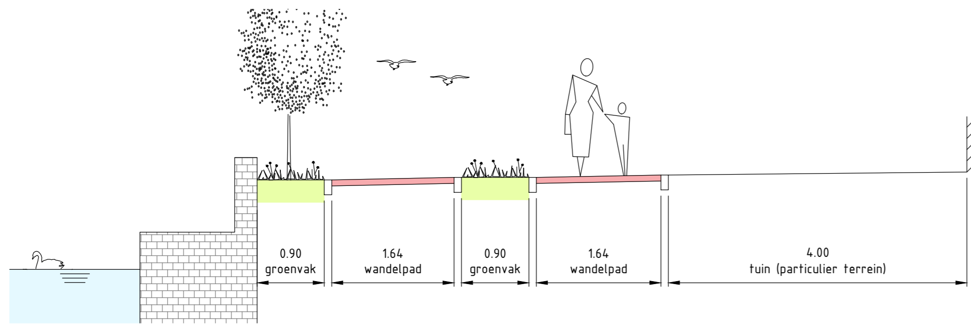
Principe profiel herinrichting Wipmolen Schaal 1:50
