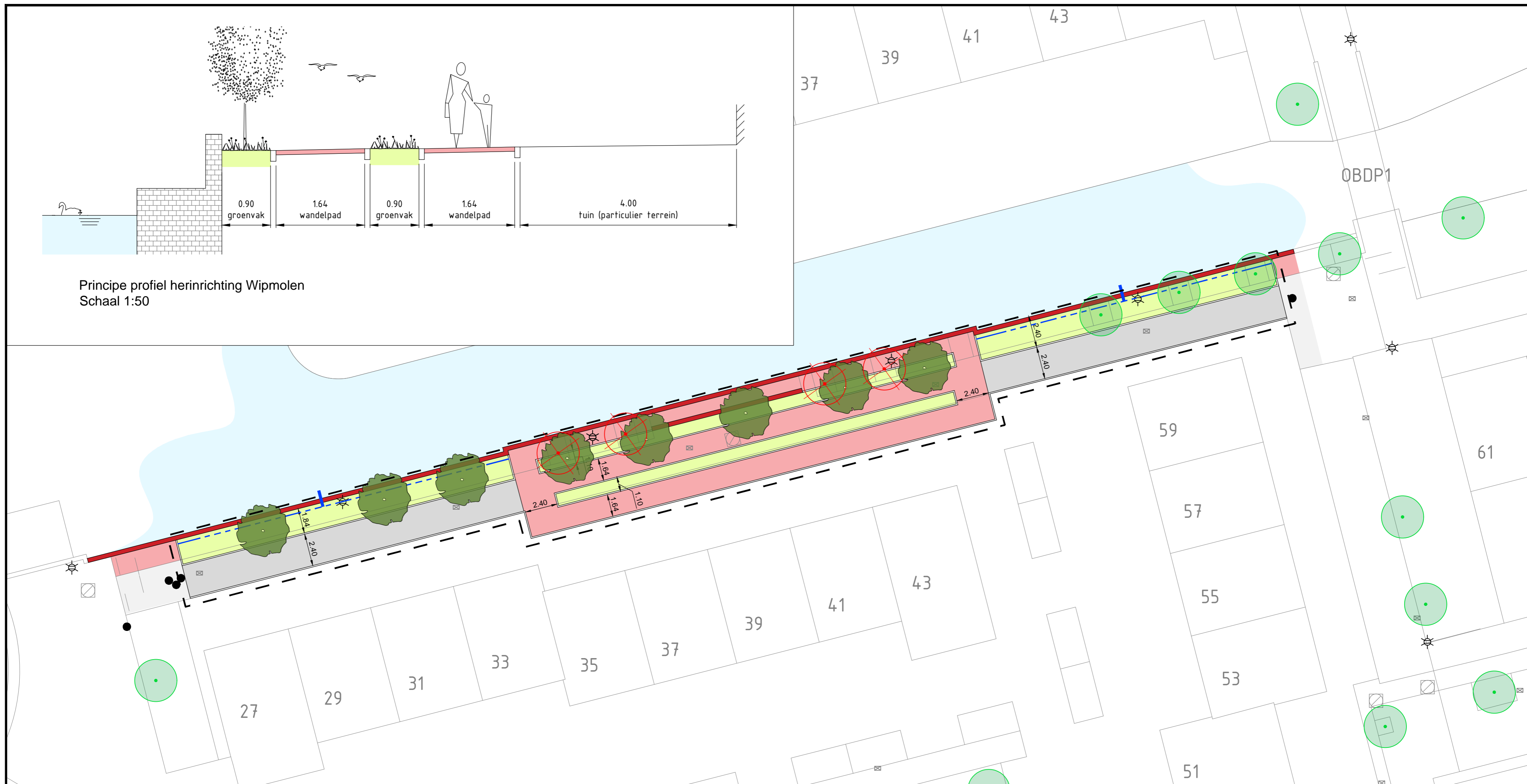
Overzichtstekening Wipmolen Schaal 1:200
