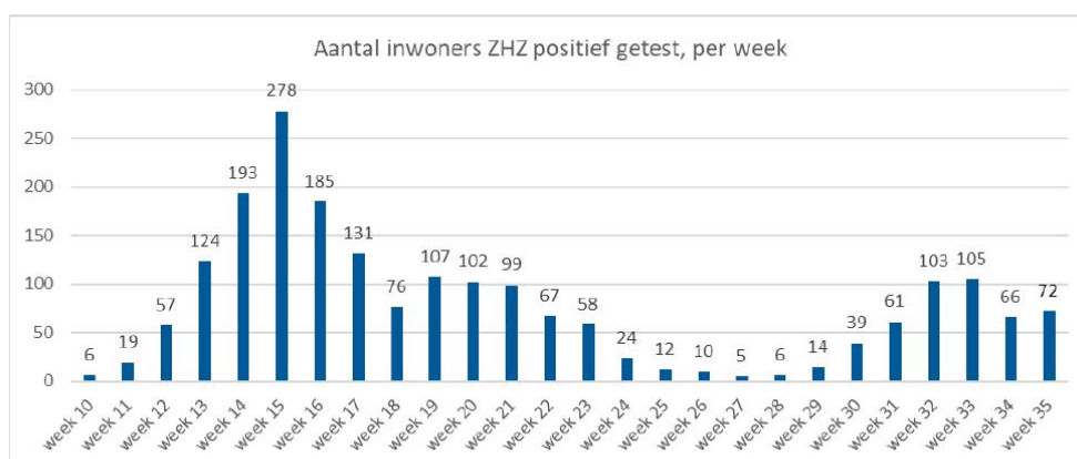
Grafiek 1: Aantal positieve tests COVID-19 bij inwoners ZHZ, per week
